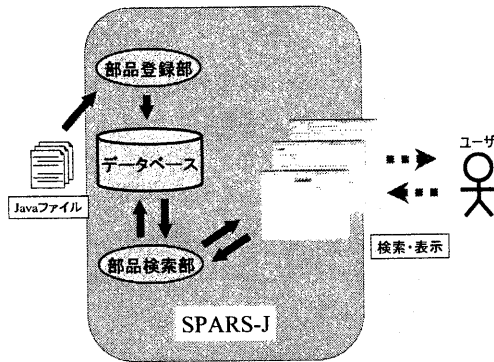
図 1 SPARS-J の構成
